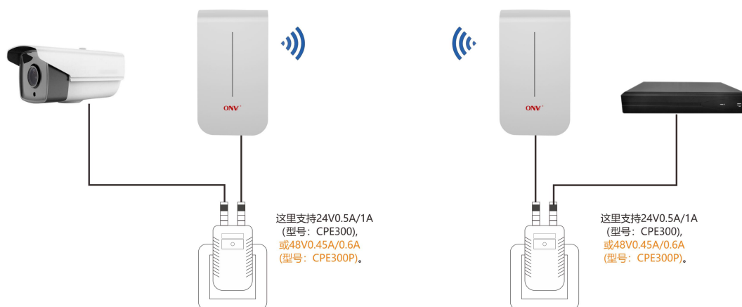
无线网桥---供电---摄像头
