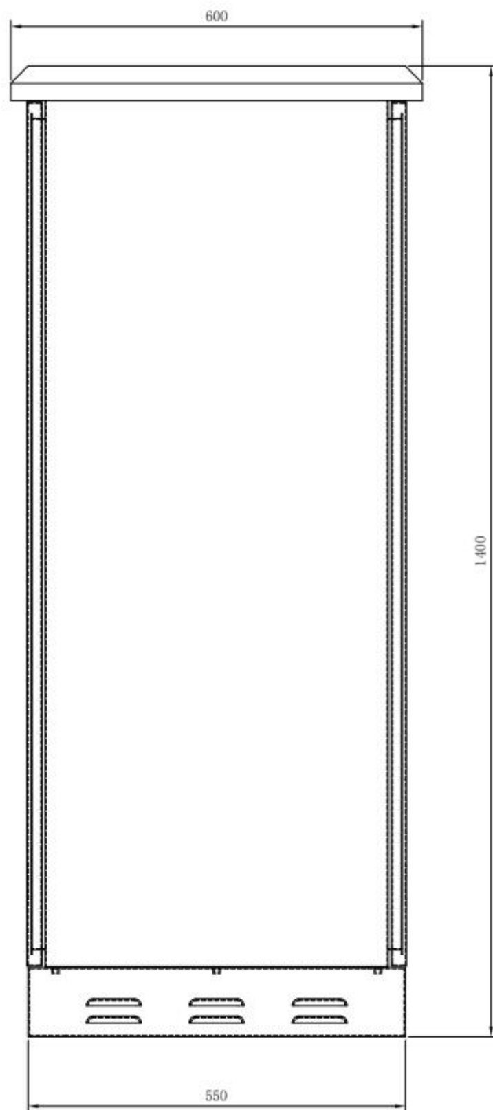
侧视图
