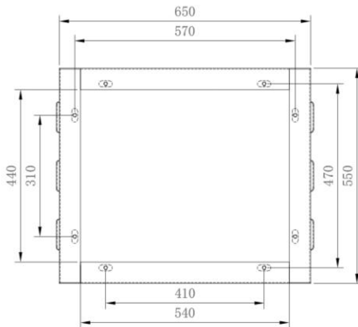
底 座 (地 笼 侧)
